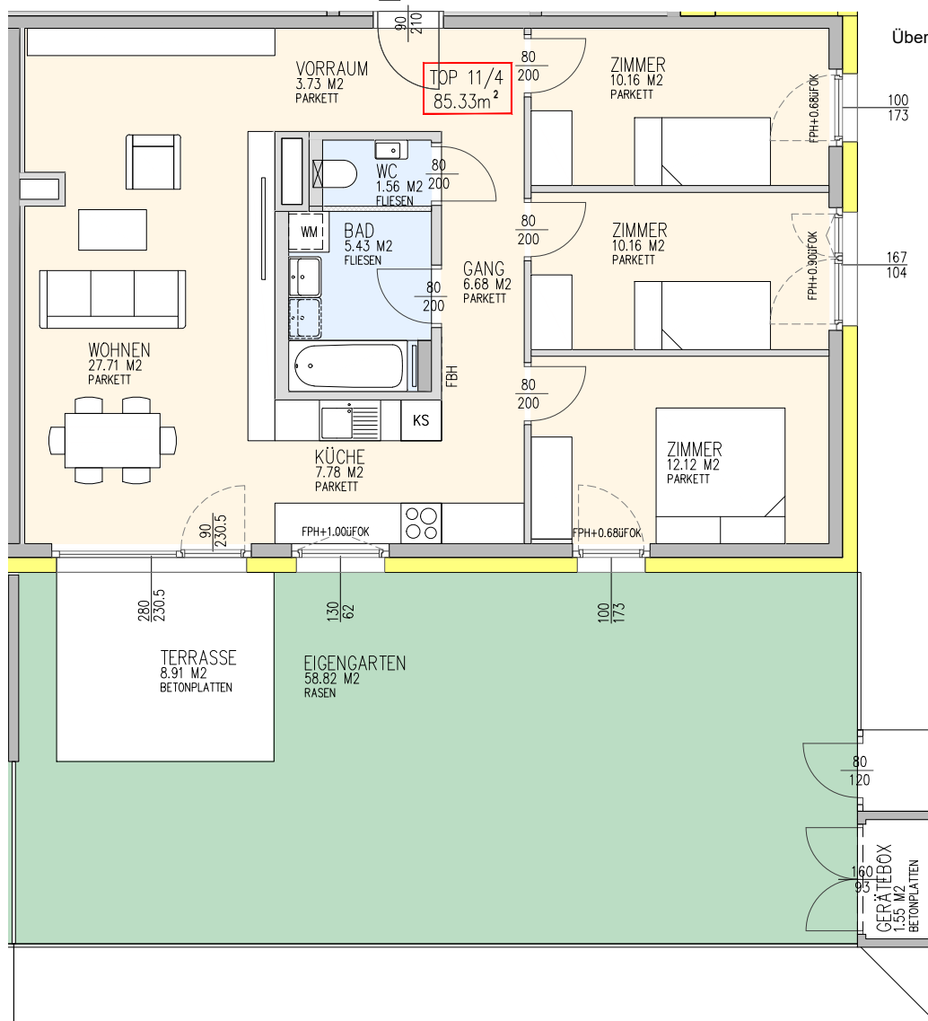
Stiege 11
