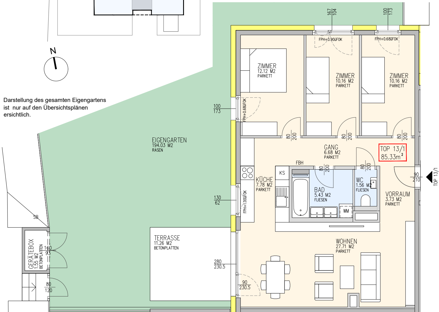
Stiege 13
