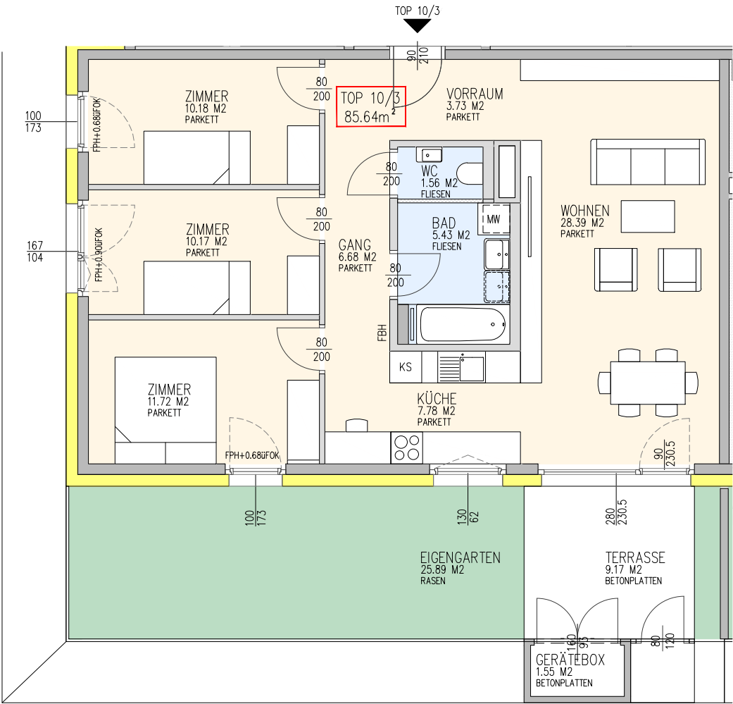
Stiege 10
