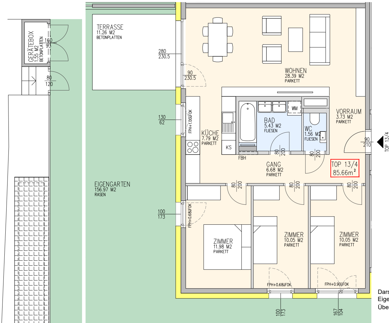
Stiege 13
