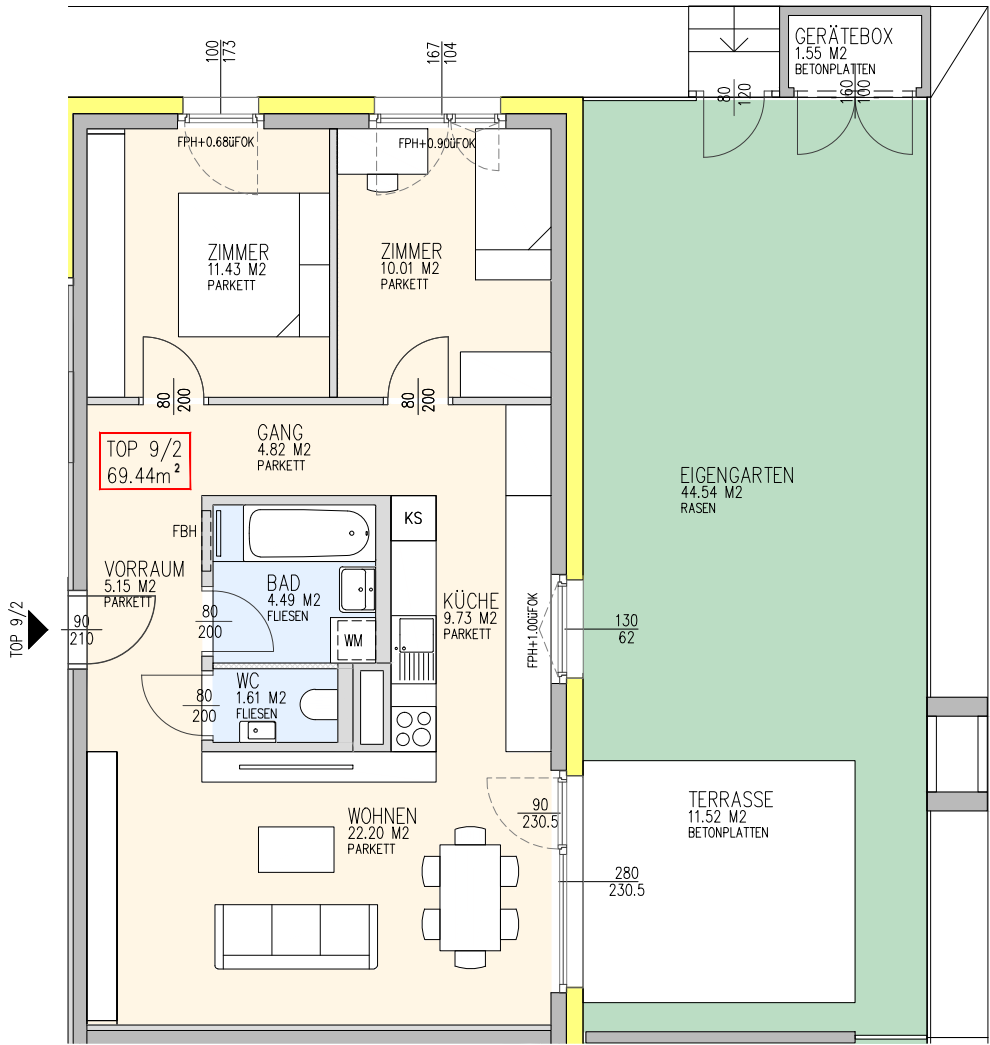
Übersicht EG
