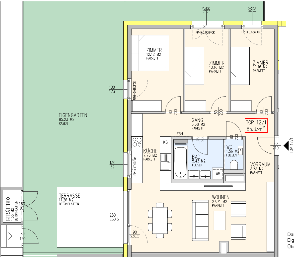
Stiege 12
