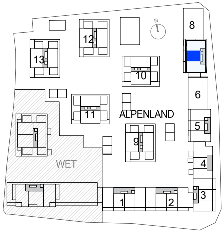
Übersicht OG4
