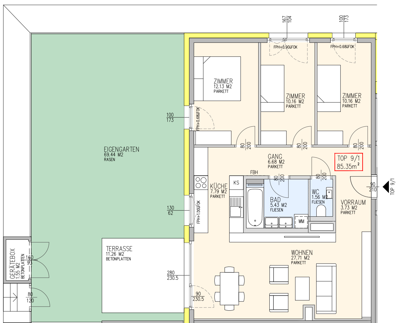
Stiege 9
