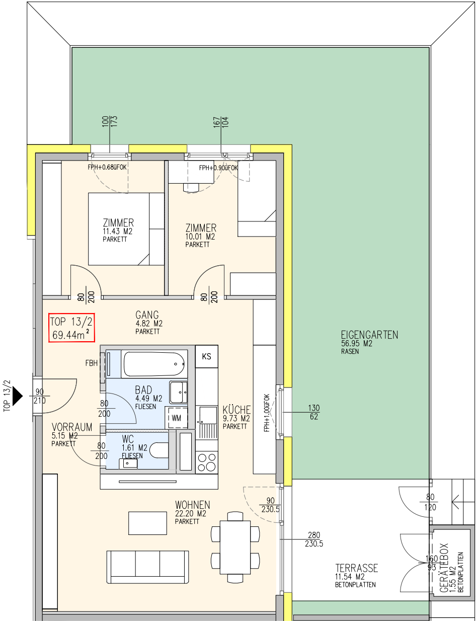
Übersicht EG
