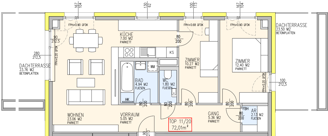
TOP 11/20
