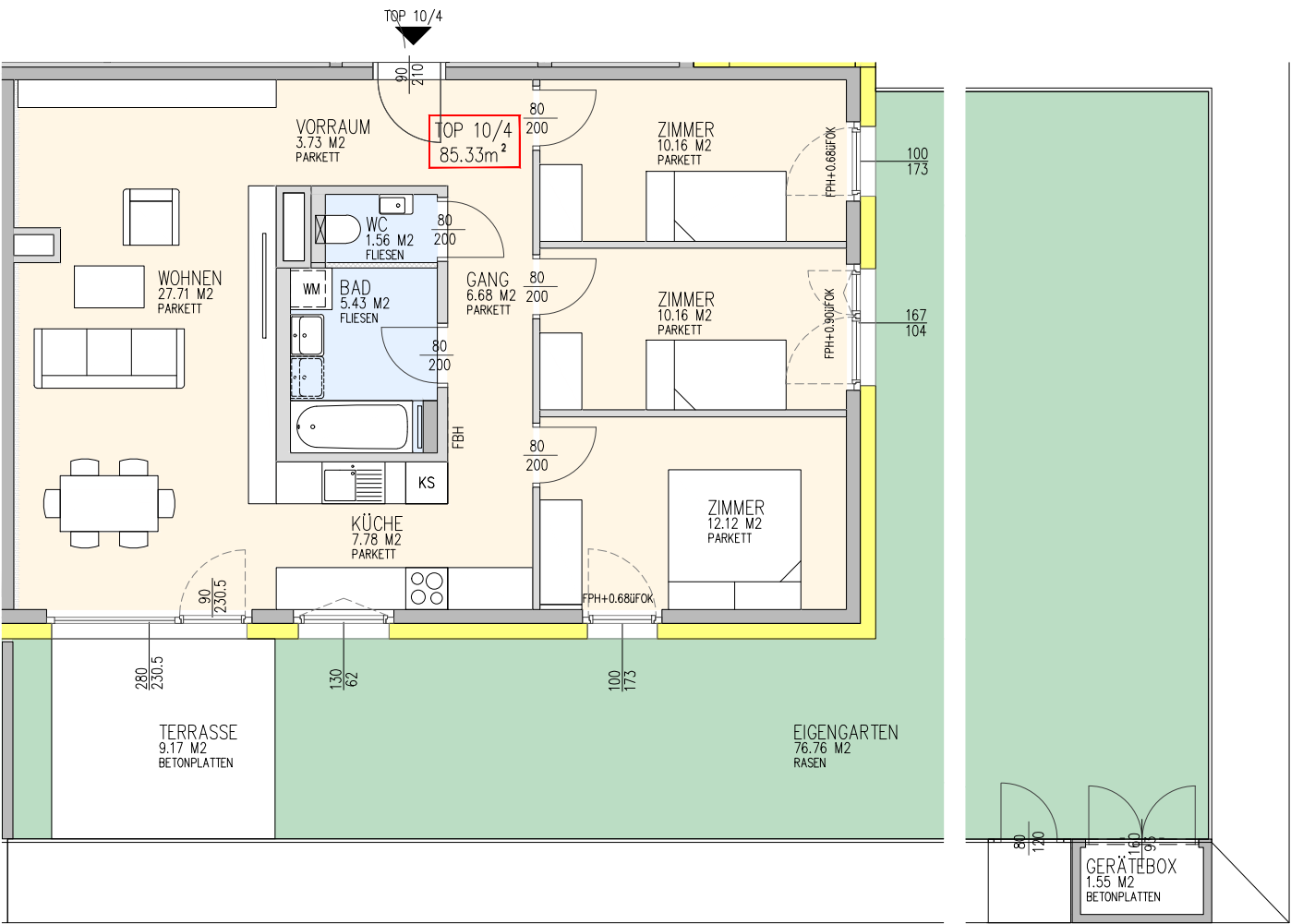
Übersicht EG 10
