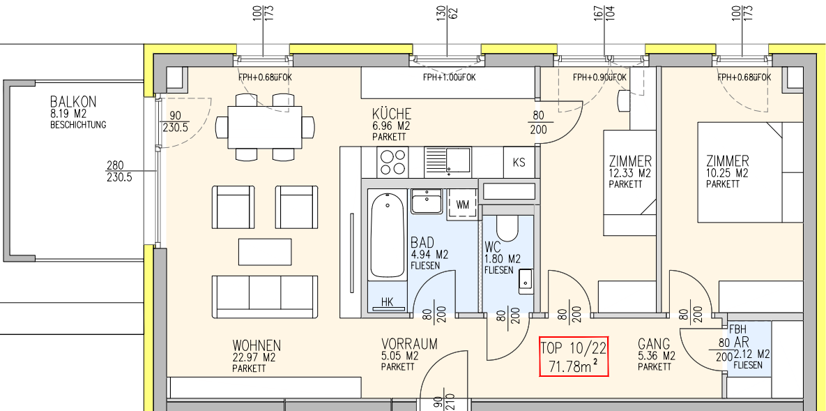
TOP 10/22
